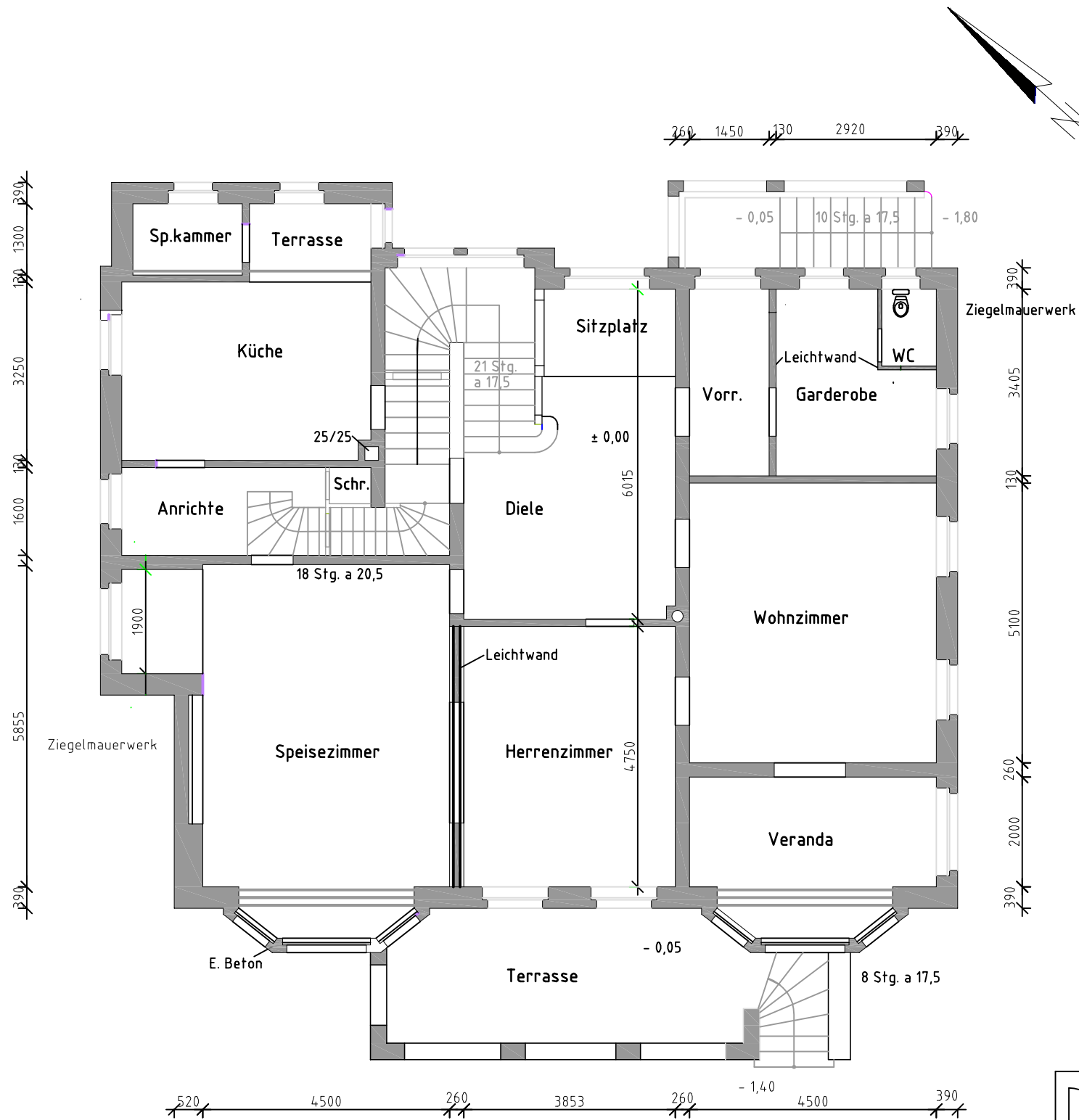
Erdgeschoss
